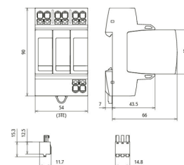
Maßbild DG MP TNC 150 FM
