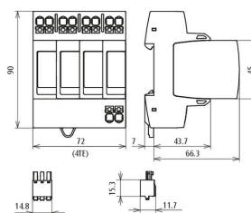
Maßbild DG MP TNS 385 FM
