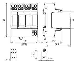
Maßbild DG MP TT 385 FM
