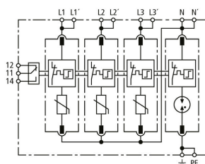
Prinzipialschaltbild DG MP TT 385 FM
