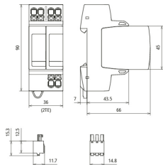
Maßbild DG MP TN 150 FM
