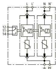
Prinzipialschaltbild DG MP TN 275 FM
