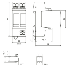
Maßbild DG MP TT 2P 275 FM
