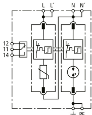
Prinzipialschaltbild DG MP TT 2P 275 FM
