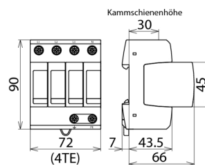
Maßbild DG M TNS 385
