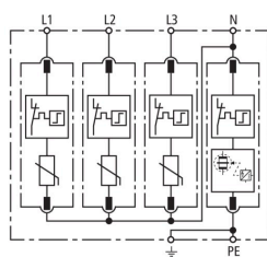
Prinzipschaltbild DG M H TT 275
