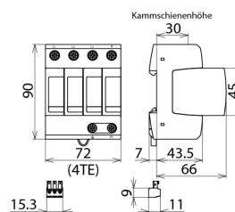
Maßbild DG M TT 320 FM
