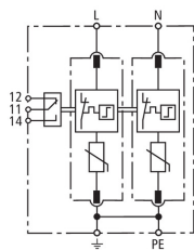
Prinzip Schaltbild DG M TN 275 FM
