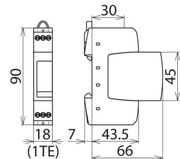
Maßbild DR M 2P 75
