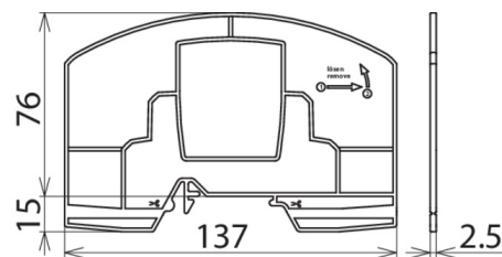
Maßbild Trennwand
