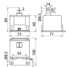
Maßbild DBM 1 255 S
