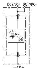
Principalschaltbild DSE M 1 60
