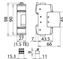
Maßbild DG SE DC 242 FM
