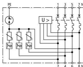
Prinzip Schaltbild SPD+POP 4 255 C32
