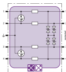
Prinzipialschaltbild BXT ML4 BC 5
