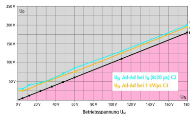
Schutzpegeldiagramm DBX U4 KT BD S 0-180
