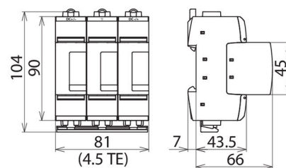
Maßbild DG ME YPV SCI 1500
