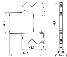
Maßbild BCO ML2 BD 12
