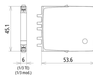
Maßbild BCO MOD ML2 BD HC5 A 24
