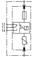
Principalschaltbild DG MOD E CI WE 440
