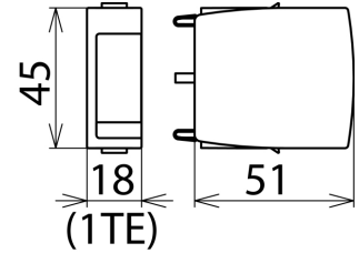
Maßbild DG MOD 600
