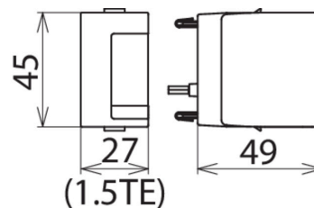
Maßbild DG MOD E PV SCI 750
