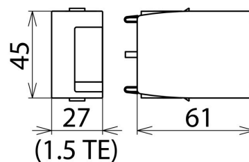
Maßbild DG MOD E H 1000 VA
