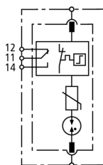
Principalschaltbild DG MOD E H 1000 VA
