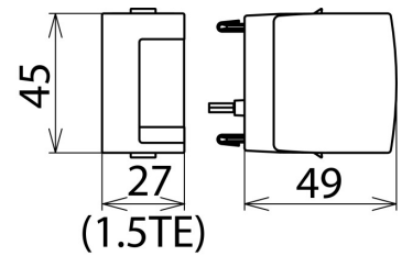
Maßbild DG MOD E DC 60
