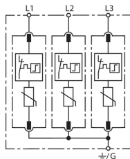
Prinzipialschaltbild DG MU 3PY 208 3W+G
