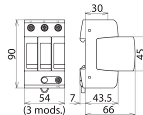
Maßbild DG MU 3PY 208 3W+G
