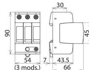
Maßbild DG MU 3PY 600 3W+G
