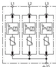
Prinzipialschaltbild DG MU 3PY 600 3W+G
