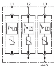
Prinzipialschaltbild DG MU 3PD 480 3W+G
