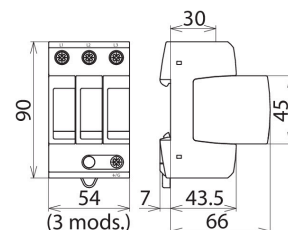
Maßbild DG MU 3PD 480 3W+G
