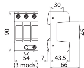
Maßbild DG MU 3PD 240 3W+G
