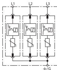
Prinzipialschaltbild DG MU 3PD 240 3W+G
