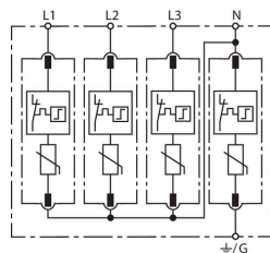
Prinzip Schaltbild DG MU 3PY 208 4W+G
