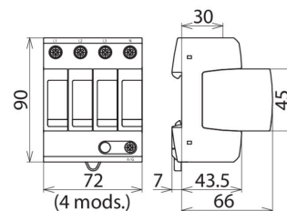
Maßbild DG MU 3PY 208 4W+G
