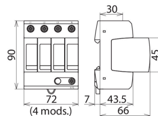
Maßbild DG MU 3PY 600 4W+G
