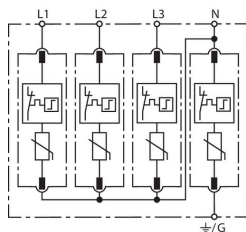
Prinzipialschaltbild DG MU 3PY 600 4W+G
