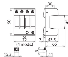
Maßbild DG MU 3PY 480 4W+G R
