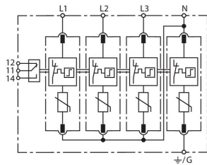
Prinzipialschaltbild DG MU 3PY 480 4W+G R
