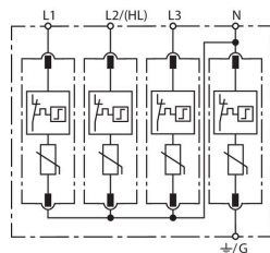
Prinzip Schaltbild DG MU 3PH 240 4W+G
