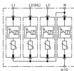
Prinzip Schaltbild DG MU 3PH 480 4W+G
