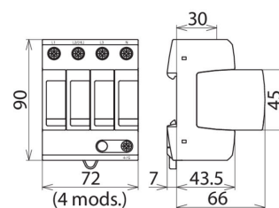
Maßbild DG MU 3PH 480 4W+G
