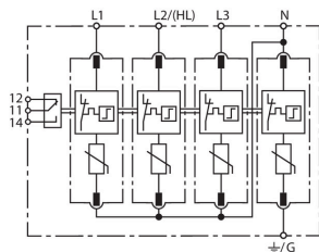
Prinzipialschaltbild DG MU 3PH 240 4W+G R
