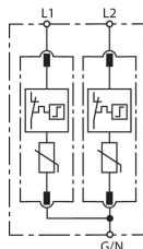
Principalschaltbild DG MU SP 480 3W+G
