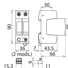
Maßbild DG MU SP 480 3W+G R
