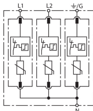
Prinzipialschaltbild DG MU 3PY 208 3W+G
