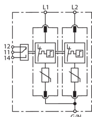
Prinzipialschaltbild DG MU CGD 240 3W+G
