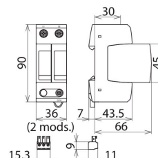
Maßbild DG MU CGD 240 3W+G
