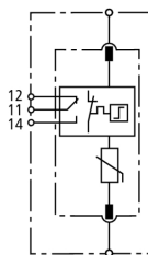
Prinzipialschaltbild DG S 150 FM
