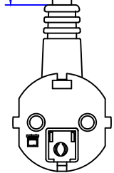
CEE7/7 Winkelstecker Typ 30D
