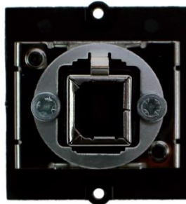
Rückansicht
