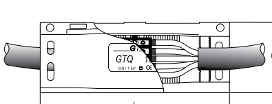
Verbindungsmuffe Typ GTQ 16L
