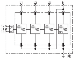
Prinzipialschaltbild DV M2 TT 255 FM
