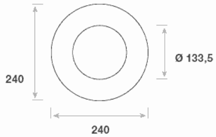
Lochblende RD-DLA1-M
