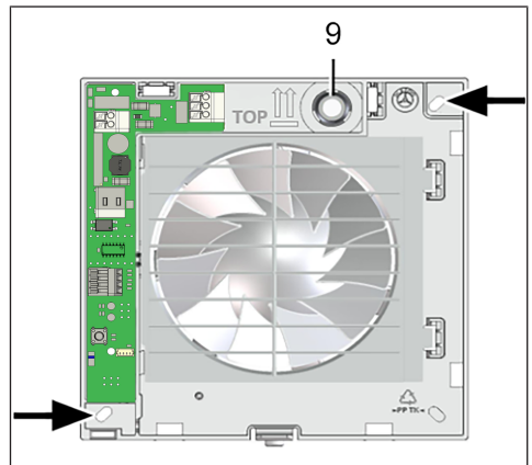
9 Cable grommet
