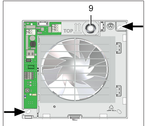
9 Leitungstülle
