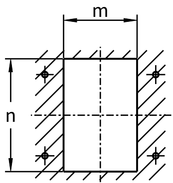
Montageausschnitt/ Mounting cutout
