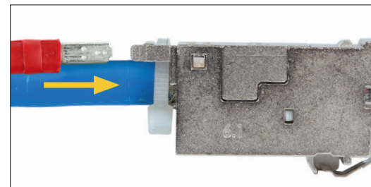
Optionaler Potentialausgleich mit 2,8 mm Flachstecker Optional potential equalisation with 2.8 mm flat plug
