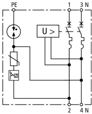
Prinzipschaltbild SPD+POP 2 255 C40
